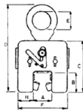
Prijemalo za tračnice tip IPRLN
