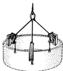
Prijemalo za jaške SRG
